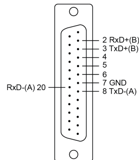
RS-422/RS-485-4w
