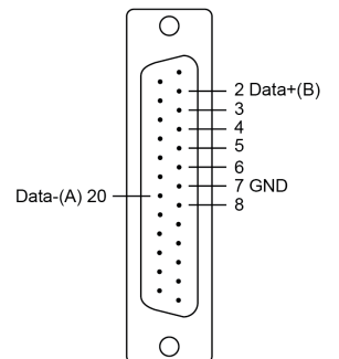
RS-485-2w
