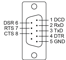
RS-232
