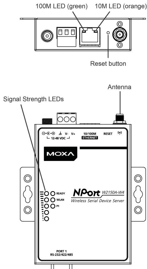
NPort W2150A-W4/W2150A-W4-T
