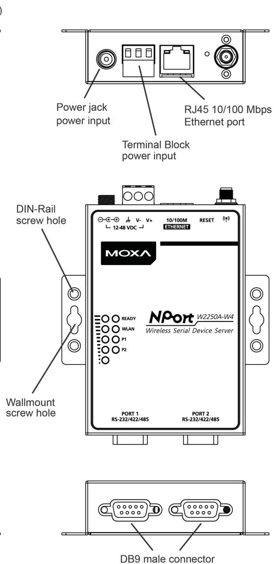
NPort W2250A-W4/W2250A-W4-T
