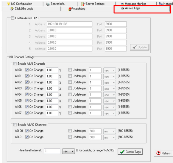
ioLogik E2240
