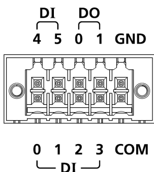
DIs x 6 / DOs x 2 (Terminal Block)
