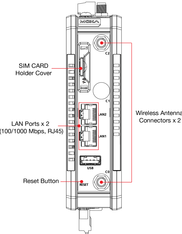
CCG-1520 前視圖
