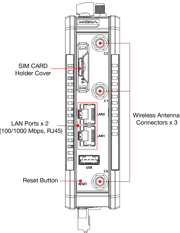
CCG-1520 前視圖
